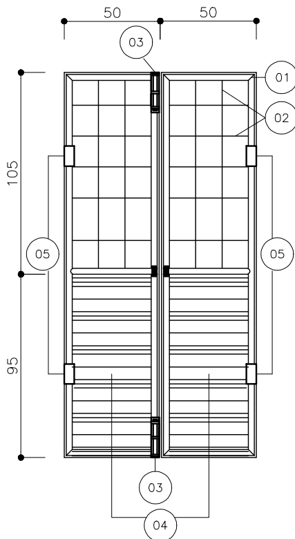
DETALHE - PORTA
